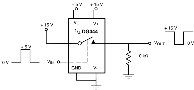
Fig. 7 - Level Shifter
