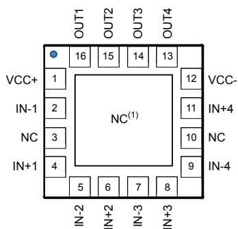
QFN16 3x3
