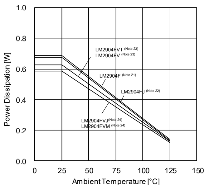
(d) LM2904xxx
