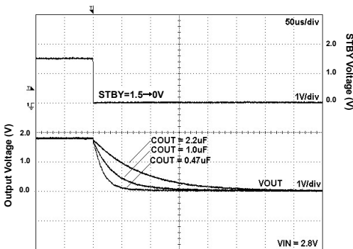
Fig 26. Discharge Time
