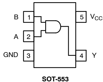
SOT-553
