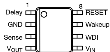
SO-8 EP
