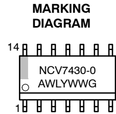
SOIC-14 D2 SUFFIX CASE 751A
