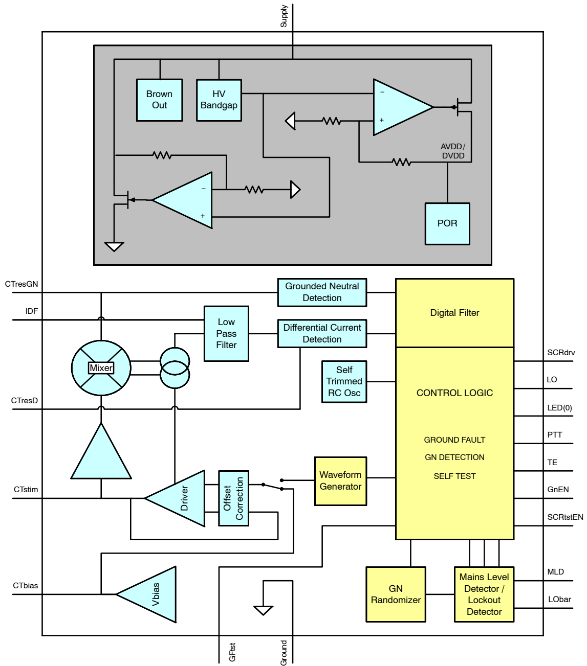
GFCI ASIC
