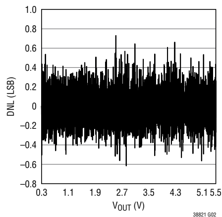
VOUT_COMMAND DNL
