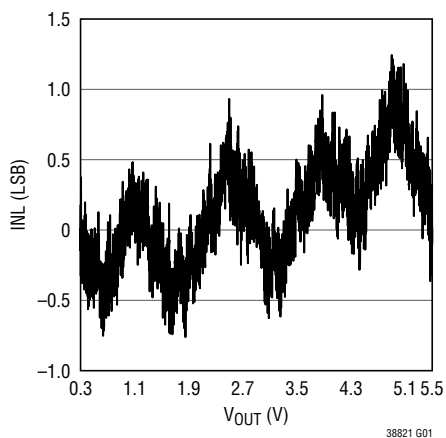
VOUT_COMMAND INL
